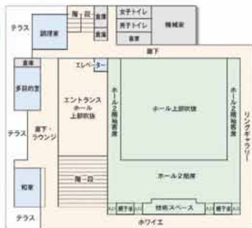
平面図 2階
