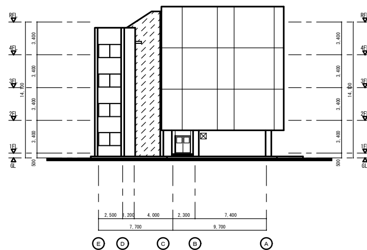
南側立面図 S=1/200
