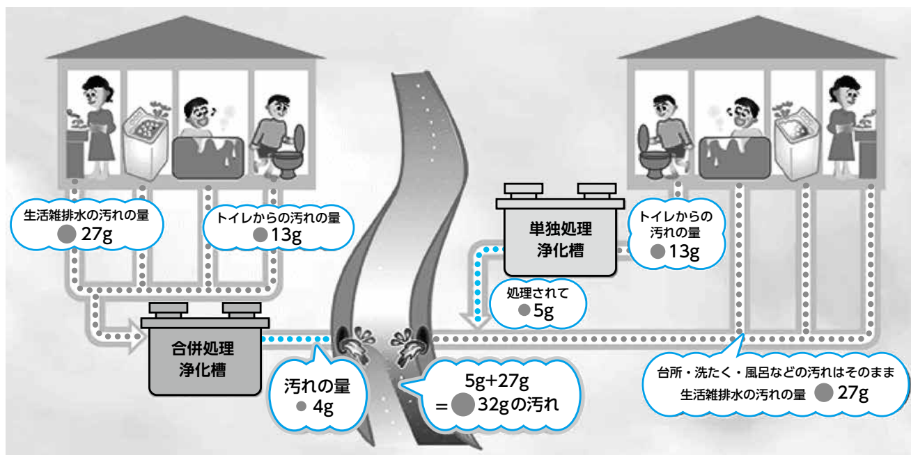
合併処理浄化槽と単独処理浄化槽の違い (千葉県浄化槽検査センターホームページより)
