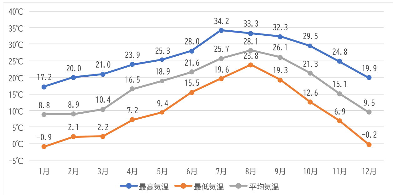
図1－3 気温の経月変化（2024（令和6）年）
