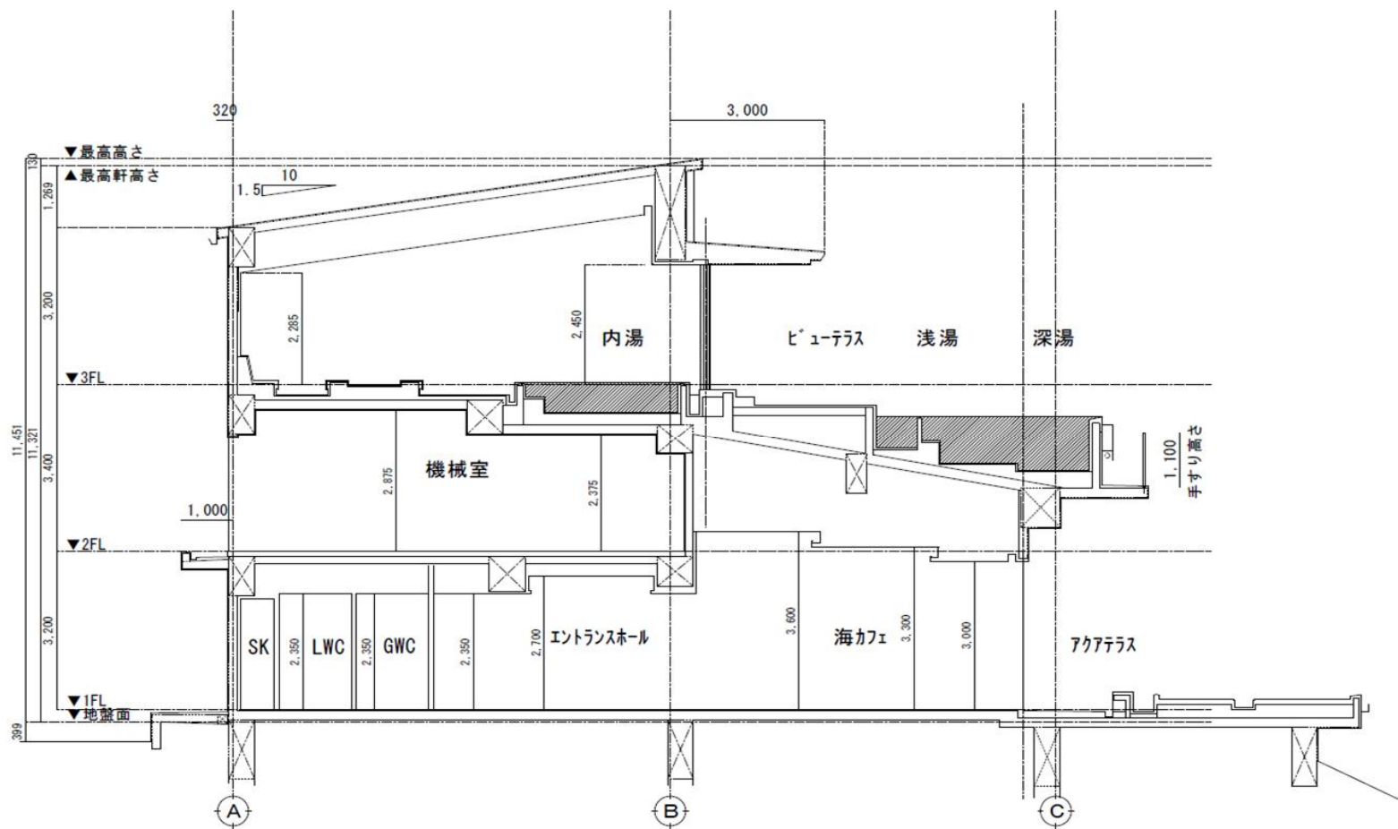
南北断面図 S=1:100
