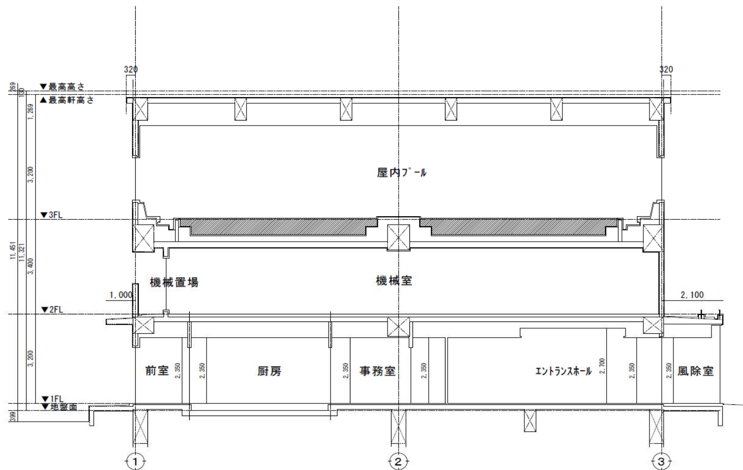
東西断面図 S=1:100
